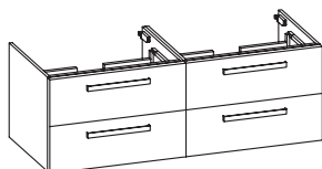
Waschtischunterschrank mit Siphonausschnitt 4 Auszüge
