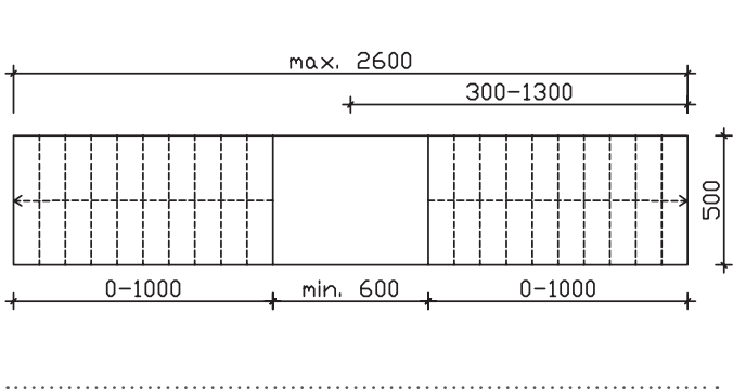
Breite 600-2600 mm KVS152650H-_____
